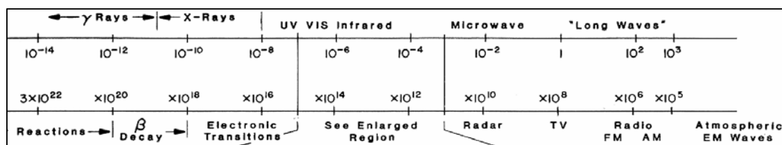
Fig 1: Het elektromagnetisch spectrum omvat een zeer grote range van stralingstypen variërend van de hoogerenergetische gammastraling tot de zeer langgolvlige radargolven. De lengte is weergegeven in meters.
